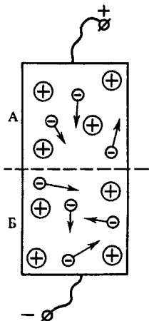
Заряды областей A и B не равны из-за хаотического движения носителей
