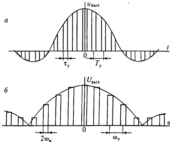
Рис. 12.2. Стробирование идеального низкочастотного сигнала: а — временная диаграмма сигнала на выходе стробирующего устройства; б — спектральная плотность выходного сигнала
