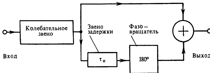
Рис. 16.5. Структурная схема согласованного фильтра для прямоугольного радиоимпульса
