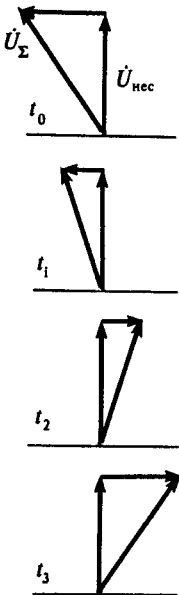
Векторные диа- граммы сигнала с угловой модуляци- ей в четыре после- довательные мо- мента времени
