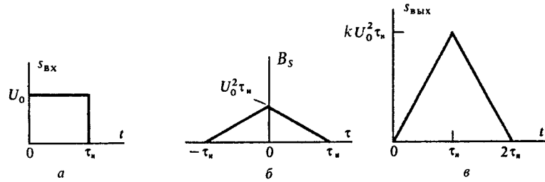
Рис. 16.2. Построение сигнала на выходе фильтра, согласованного с прямоугольным видеоимпульсом:
