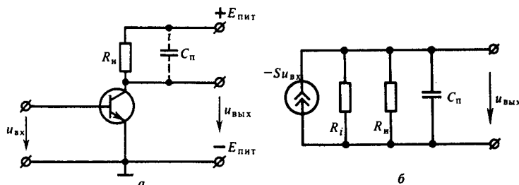
Рис. 8.1. Усилитель напряжения:
