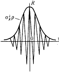
Типичная функция корреляции узкополосного случайного процесса
