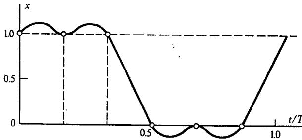
Рис. 15.5. Сигнал, восстановленный по коэффициентам ДПФ
