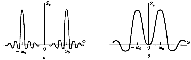
Рис. 2.9. Графики спектральных плотностей радиопульса с прямоугольной огибающей:
