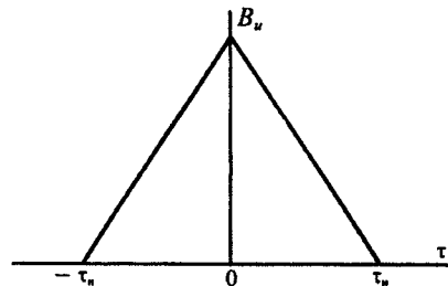
Рис. 3.4. Нахождение АКФ прямоугольного видеоимпульса
