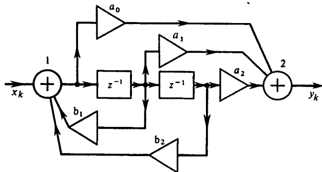
Рис. 15.10. Структурная схема канонического рекурсивного ЦФ 2-го порядка
