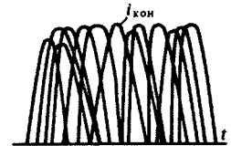
Эффект перекрытия импульсов
