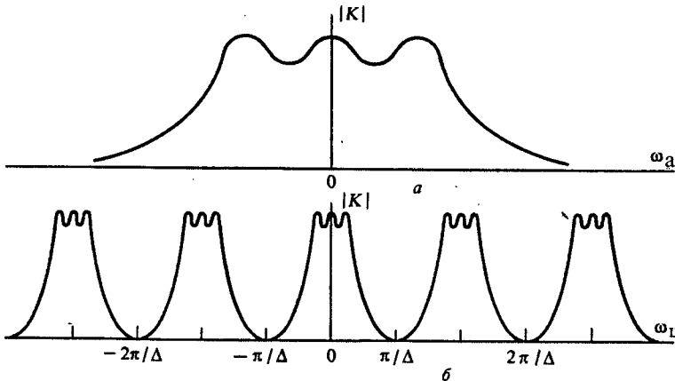
Рис. 15.12. Амплитудно-частотные характеристики фильтров: а — аналогового; б — цифрового
