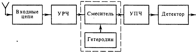
Рис. 12.1. Структурная схема супергетеродинного приемника
