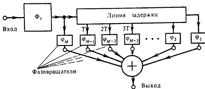
Рис. 16.6. Структурная схема согласованного фильтра для сигнала Баркера
