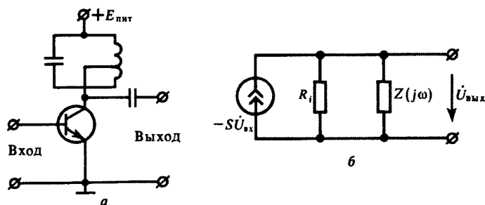
Рис. 9.2. Резонансный усилитель малых колебаний:
