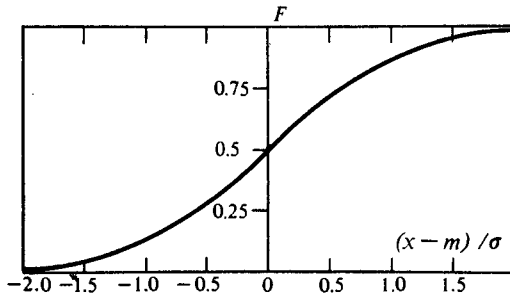
Рис. 6.2. График функции распределения гауссовской случайной величины
