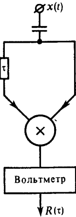
Коррелометр
