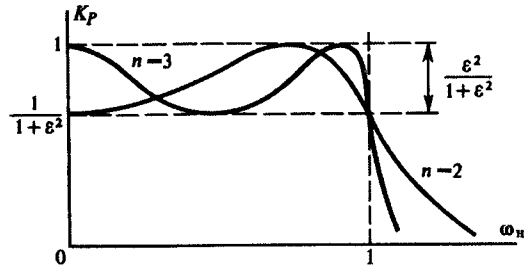
Рис. 13.3. Частотные характеристики ФНЧ чебышевского типа
