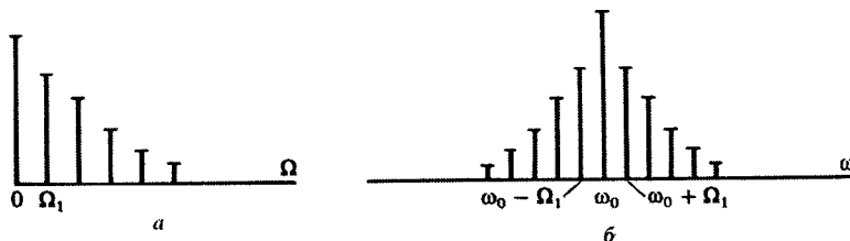
Рис. 4.2. Спектральные диаграммы:
