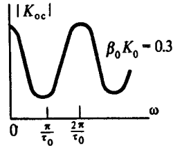
АЧХ гребенчатых фильтров
