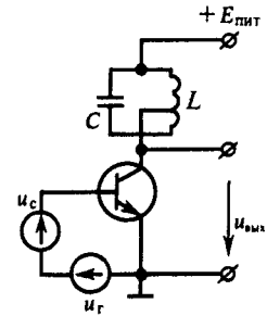
Схема преобразователя частоты
