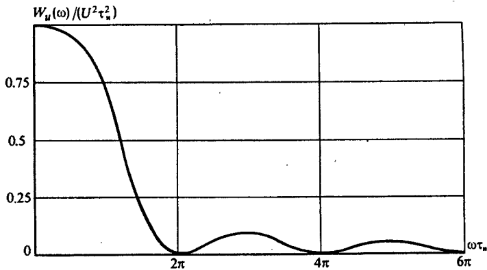
Рис. 3.2. Нормированный энергетический спектр прямоугольного видеоимпульса как функция безразмерной частотной переменной \omega\tau_u
