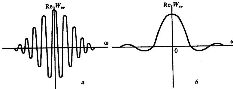
Рис. 3.1. Взаимный энергетический спектр двух экспоненциальных видеоимпульсов:
