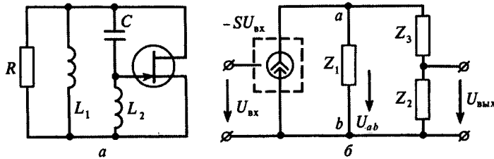
Рис. 14.12. Автогенератор по схеме индуктивной трехточки: а — принципиальная схема (источники питания и смещения не показаны); б — эквивалентная схема с разомкнутой цепью обратной связи
