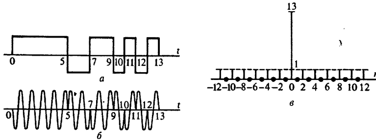
Рис. 3.7. Сигнал Баркера при M = 13 :
