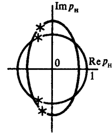
Полюсы фильтров с максимально-плоской и чебышевской характеристиками
