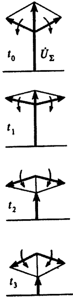
Векторные диаграммы АМ-сигнала в четыре последовательные моменты времени
