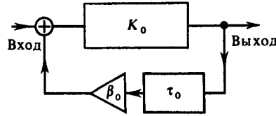
Рис. 14.4. Структурная схема системы с запаздывающей обратной связью
