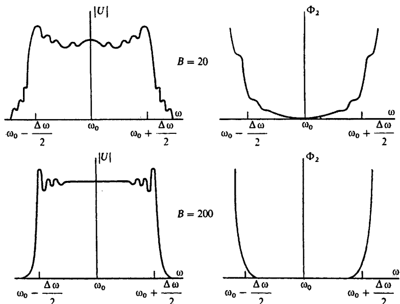
Рис. 4.10. Частотные зависимости модуля и остаточного фазового члена спектральной плотности прямоугольного ЛЧМ-импульса при различных значениях базы сигнала
