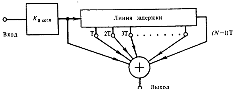
Рис. 16.4. Структурная схема согласованного фильтра для пачки видеоимпульсов
