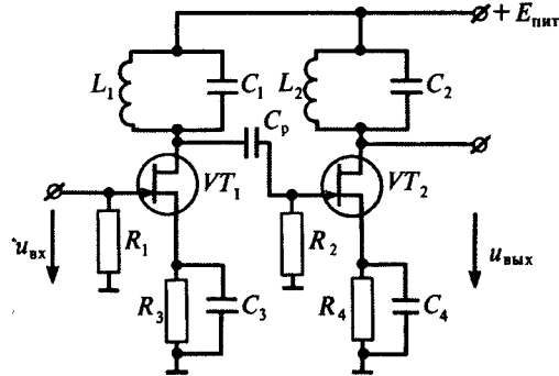
Рис. 9.4. Принципиальная схема двухконтурного усилителя
