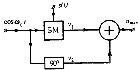
Рис. 11.10. Модулятор Армстронга
